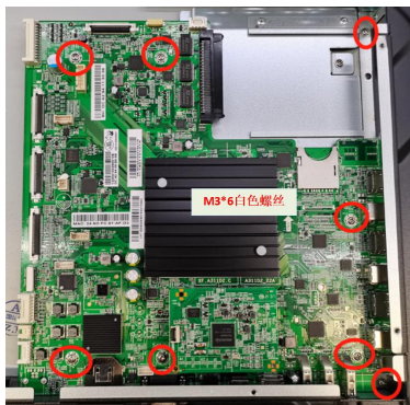
主板
